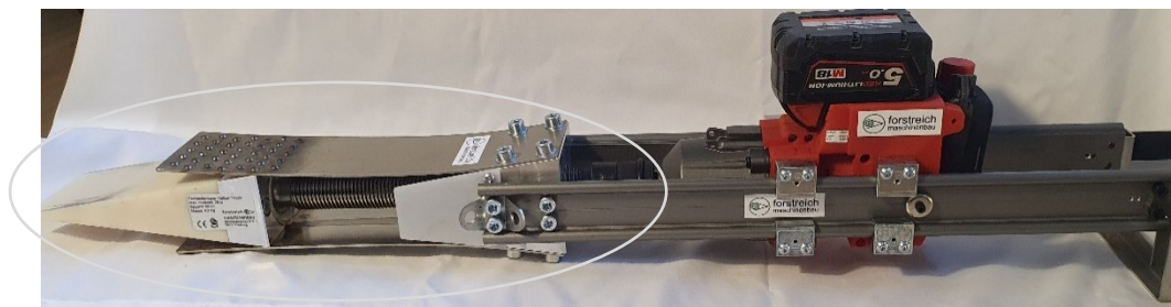
Vordere Endlage des fernbedienbaren Fällkeils – detektiert durch den Magneten auf der linken Schiene
